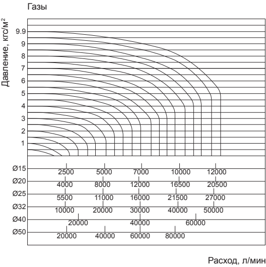
Диаграммы пропускной способности
