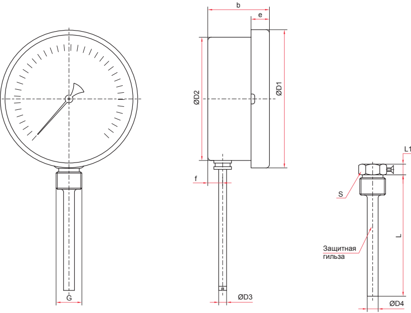
Радиальное присоединение
