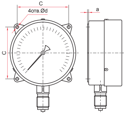
Исполнение с задним фланцем и радиальным присоединением
