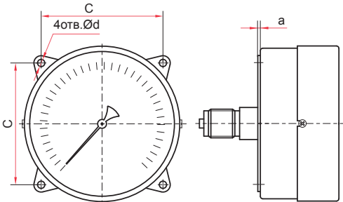
2. Осевое присоединение
